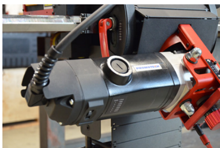
BOTTOM BEVELING
